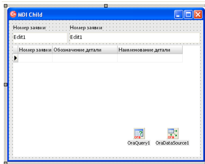
Рисунок 66. Добавление компонентов на дочернюю форму
